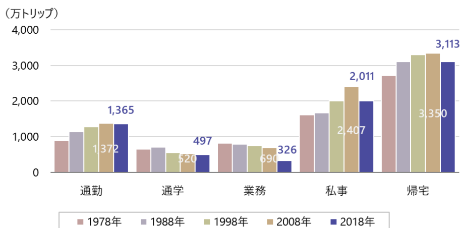
図 2-14 目的別トリップ数の推移
