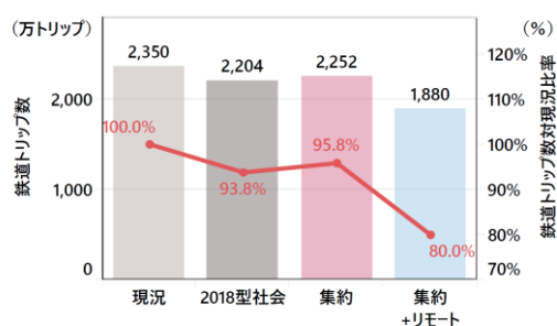
図 5-14 鉄道トリップ数の変化
