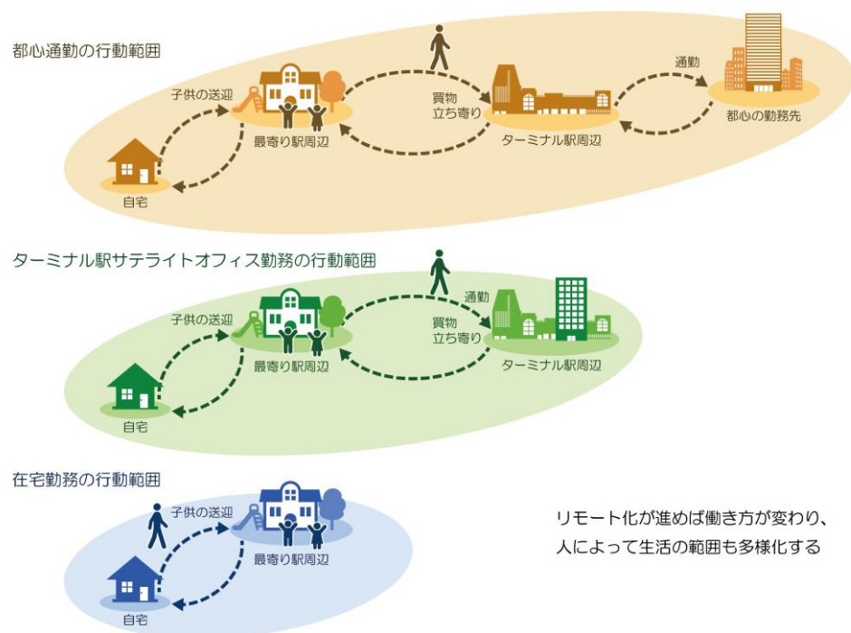
図 5-2 行動範囲のイメージ
