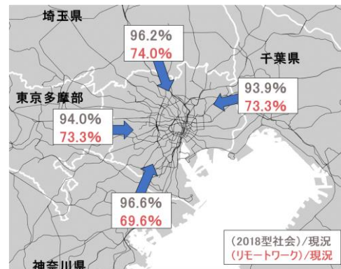
図 4-7 東京区部境界のピーク時の鉄道断面交通量の変化
