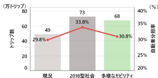
図 5-5 高齢者の自動車利用の変化
