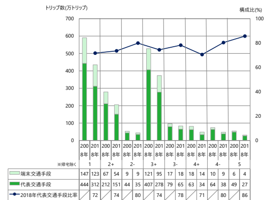
図 2-44 地域区別の自転車 トリップ数(代表+端末)
