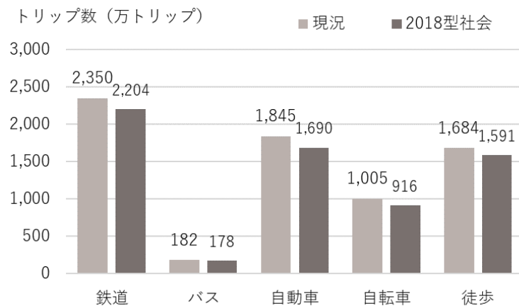
図 3-7 代表交通手段別トリップ数の変化
