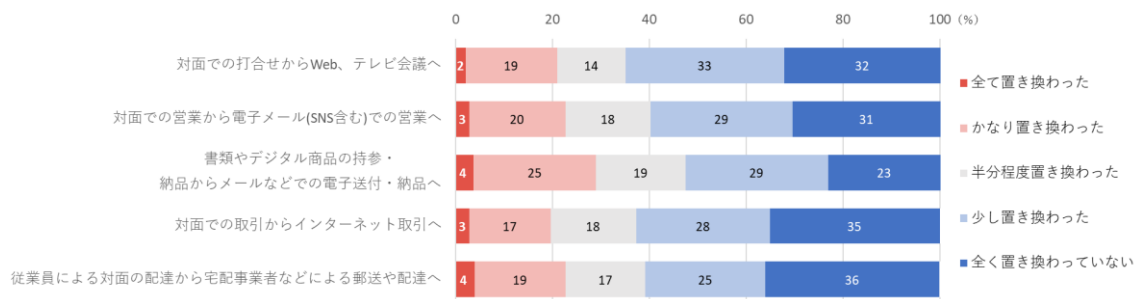
図 2-58 仕事の仕方の変化
