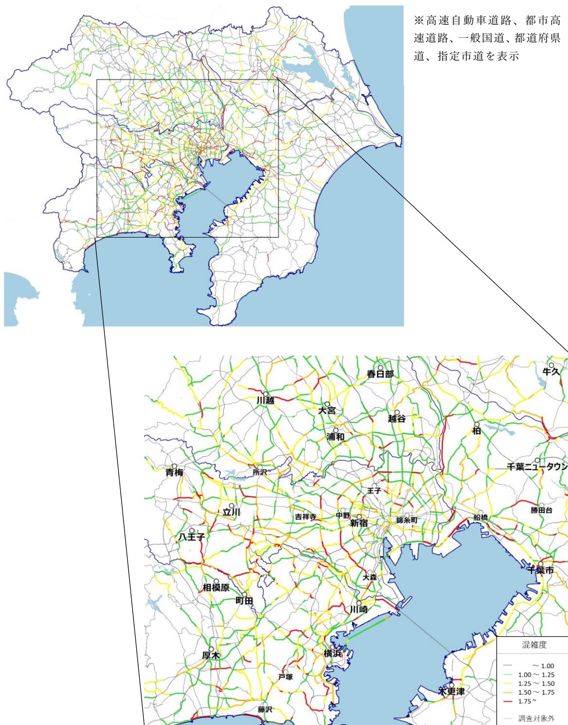
図 2-39 道路の混雑状況（平日）
