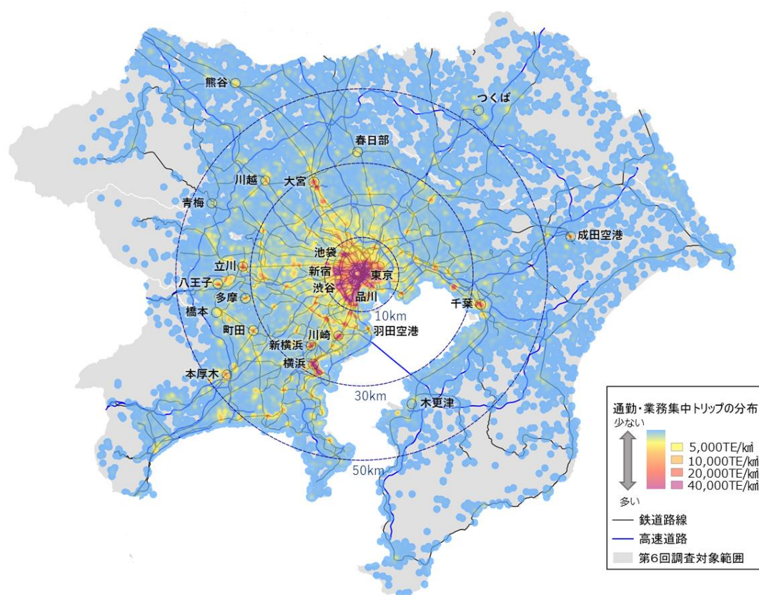
図 2-19 通勤・業務集中トリップの分布
