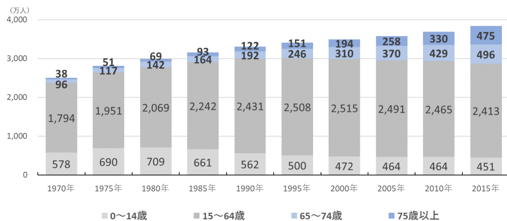
図 2-2 年齢階層別の人口の推移
