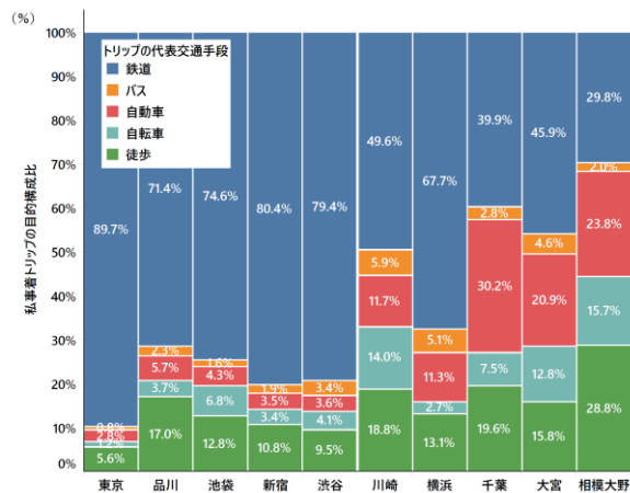
図 4-15 主要駅周辺の交通手段分担率
