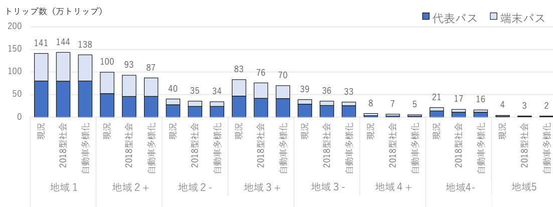
図 3-37 バストリップ数の変化
