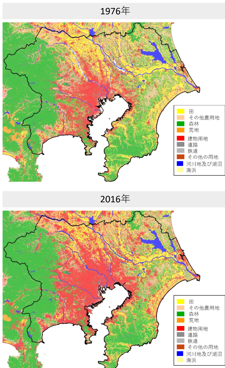
図 2-7 土地利用の変化
