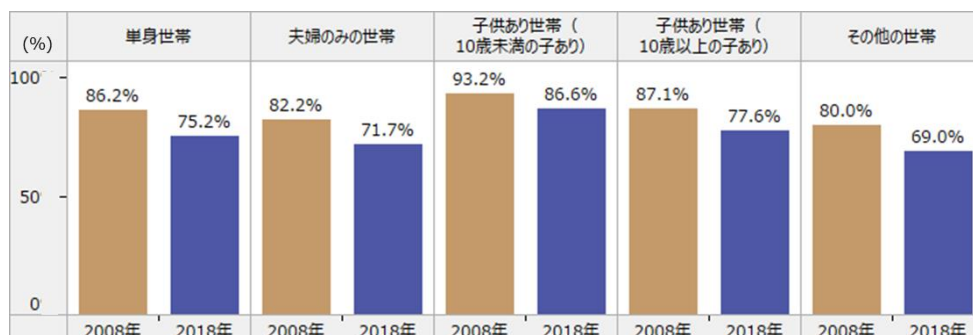
図 2-57 世帯構成別の外出率の変化
