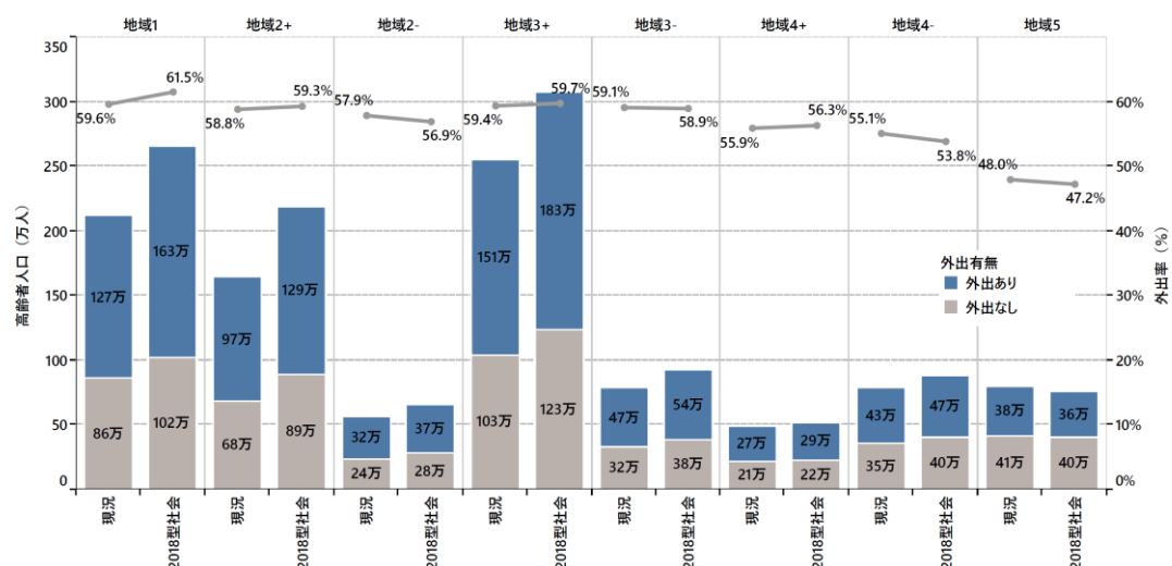
図 3-14 高齢者の外出人口と外出率の変化
