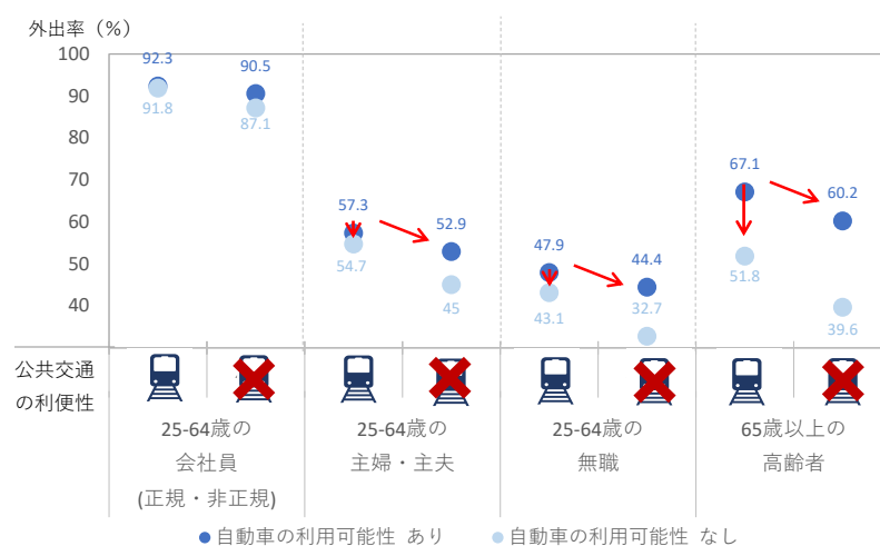
図 2-61 職業別外出率
