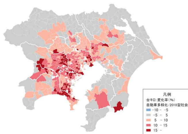
図 3-36 自動車の走行台キロの変化
