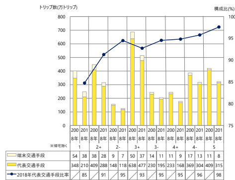
図 2-37 地域区分別の自動車トリップ数（代表＋端末）
