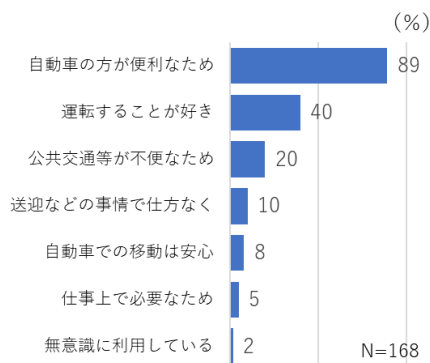
図 4-9 自動車を運転する理由
