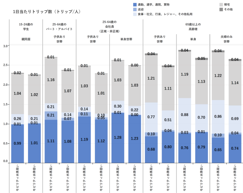
図 2-65 世帯構成別目的別の 1 人 1 日当たりトリップ数
