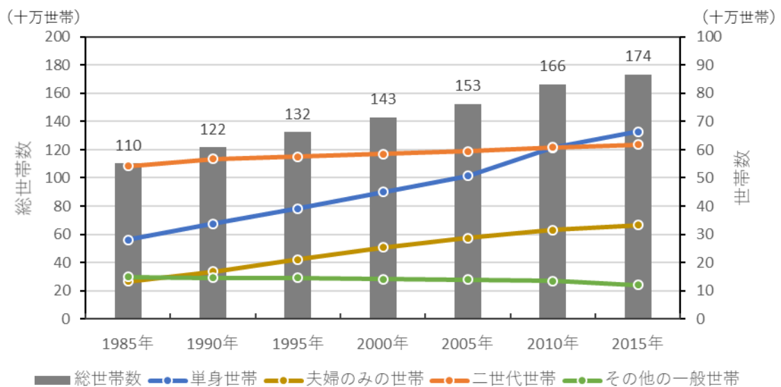
図 2-5 世帯数の推移
