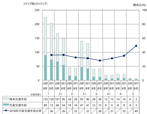
図 2-41 地域区別のバス トリップ数（代表＋端末）
