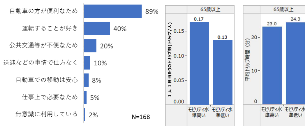
図 2-69 高齢者の自動車を運転する理由
