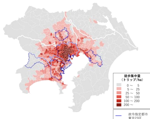
図 2-45 徒歩トリップ集中量 (端末含む)
