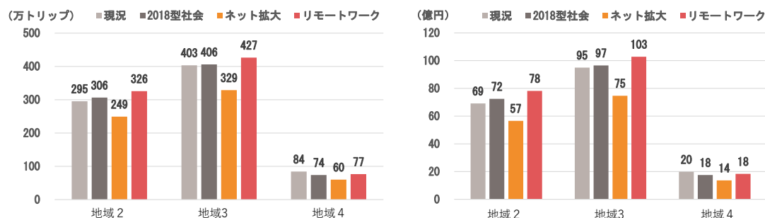
図 4-24 駅勢圏内の買物及び私事トリップ数（左）・消費金額（右）の変化
