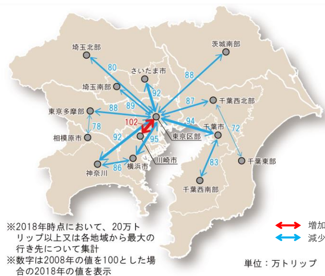
図 2-18 地域間流動の変化
