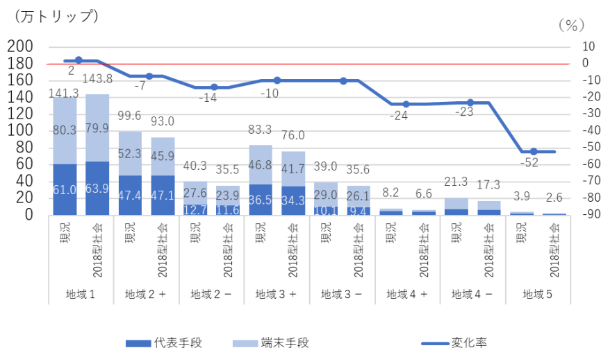
図 3-12 バストリップ数の変化
