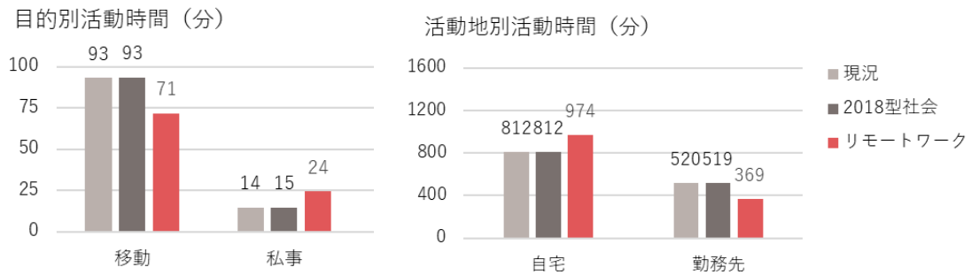
図 3-26 正規職員の一日の活動時間の変化
