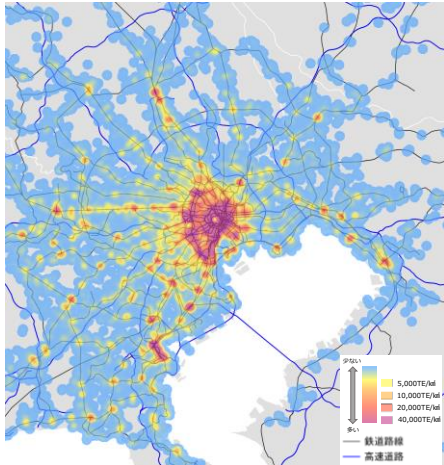
図 4-14 徒歩トリップの分布
