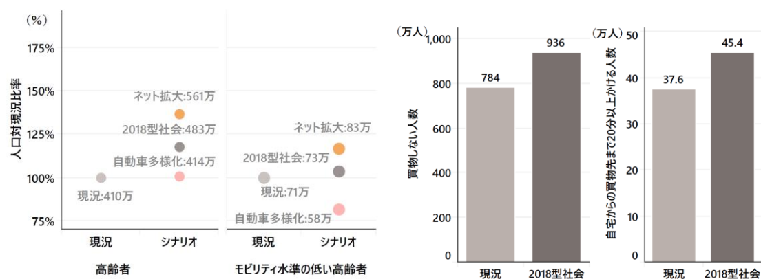
図 4-2 外出しない高齢者数の変化
