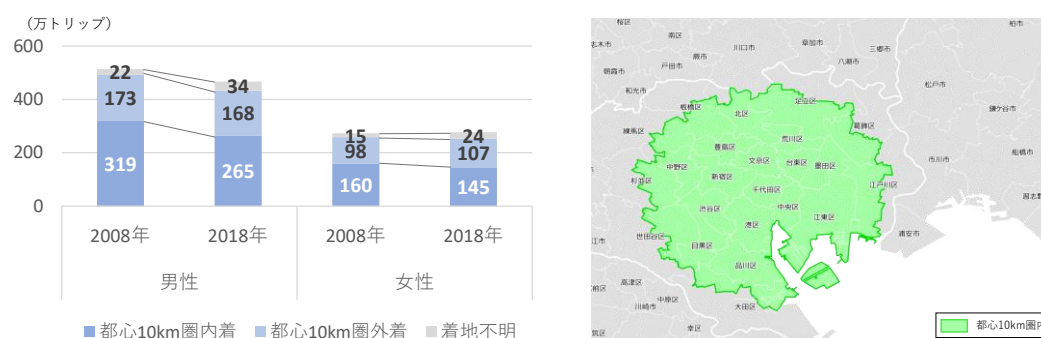
図 2-47 都心 10km 圏内、圏外への鉄道利用での通勤トリップ数の変化
