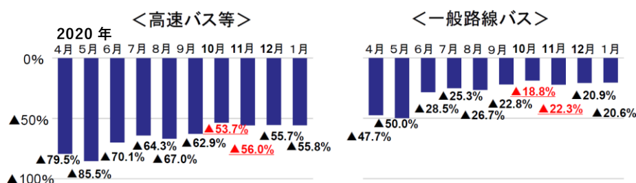
図 2-75 バスの輸送人員（前年同月比）
