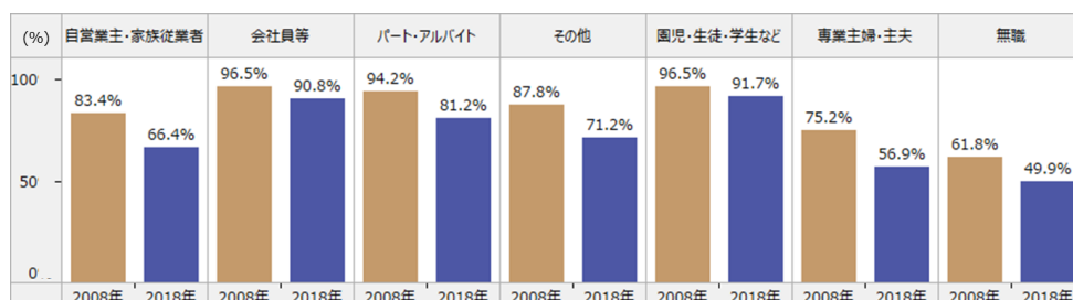
図 2-56 職業状態別の外出率の変化
