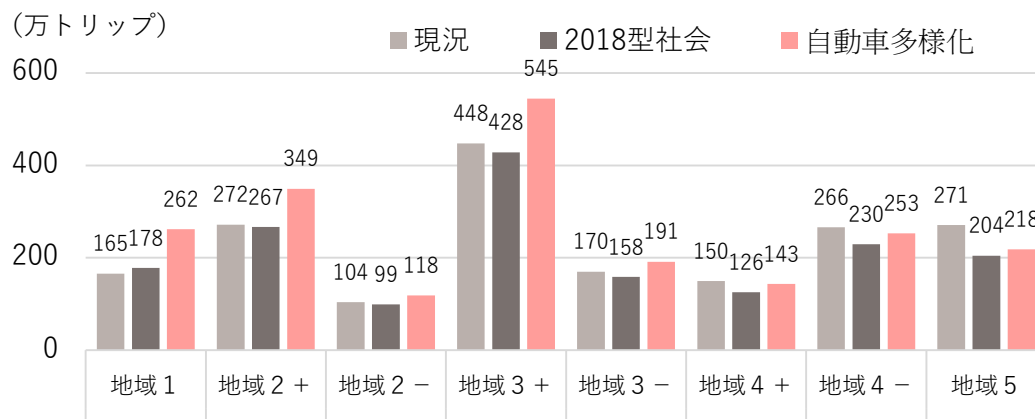
図 3-35 地域区分別の自動車トリップ数の変化
