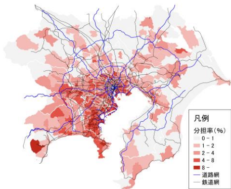
図 2-40 バス発生集中量の分担率
