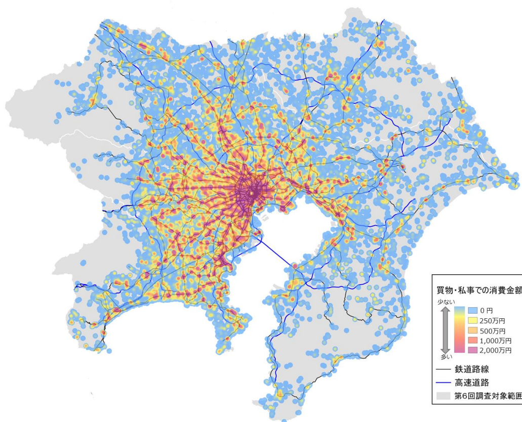
図 2-25 買物・私事での消費額の分布
