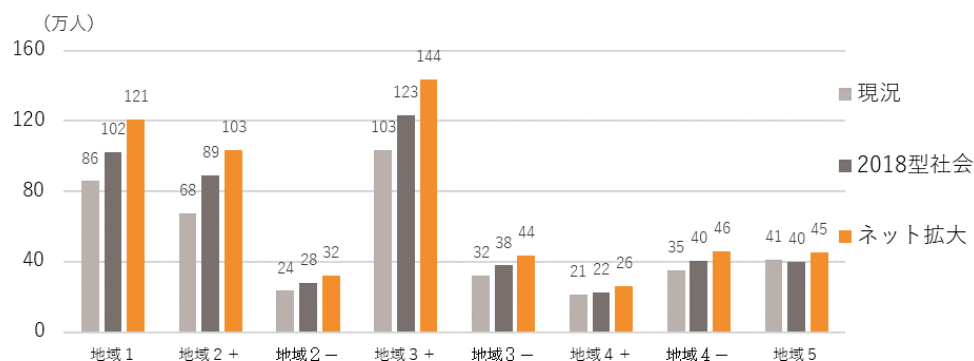
図 3-20 外出しない高齢者数の変化
