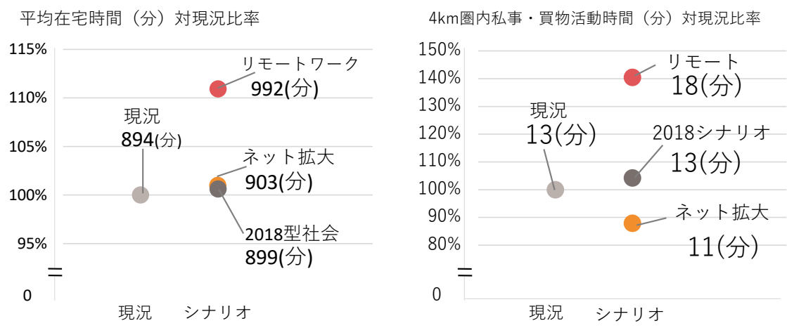
図 4-25 就業者の時間の使い方の変化
