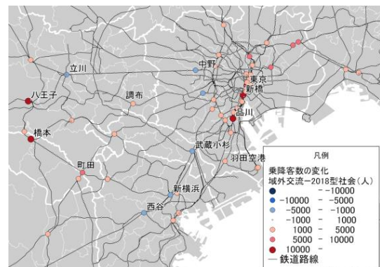
図 3-31 乗降客数の変化
