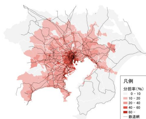
図 2-32 鉄道発生集中量の分担率
