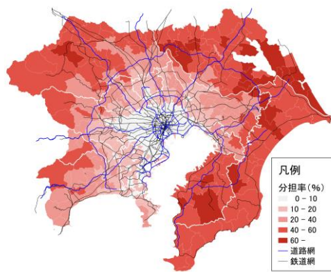
図 2-36 自動車発生集中量の分担率
