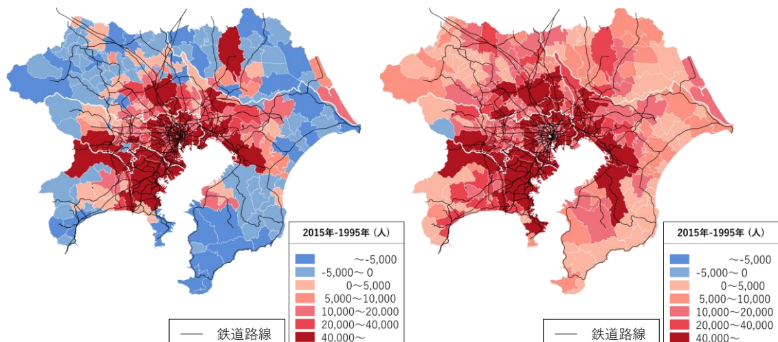
図 2-3 夜間人口分布の変化 (2015-1995)
