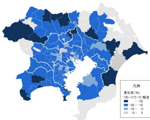
図 4-23 バストリップ数
