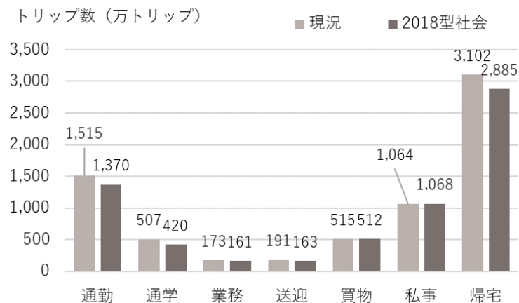
図 3-6 目的別トリップ数の変化
