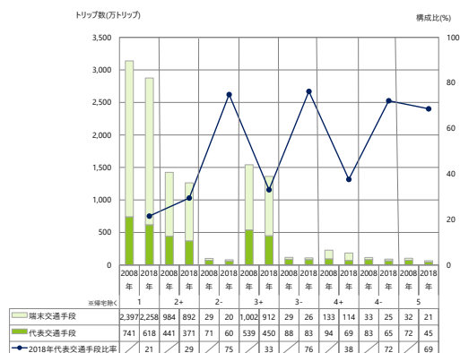
図 2-46 地域区別の徒歩 トリップ数(代表+端末)
