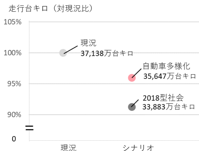
図 4-28 自動車の走行台キロの変化
