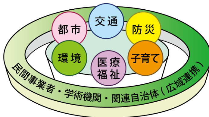
図 6-1 多様な主体との連携
