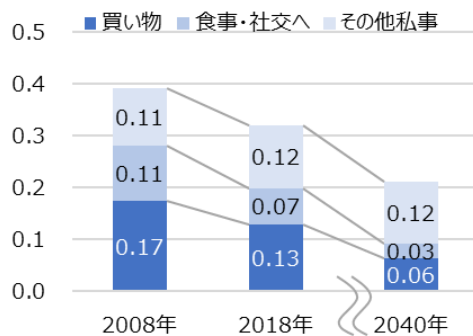
トリップ/人 非高齢者・就業
