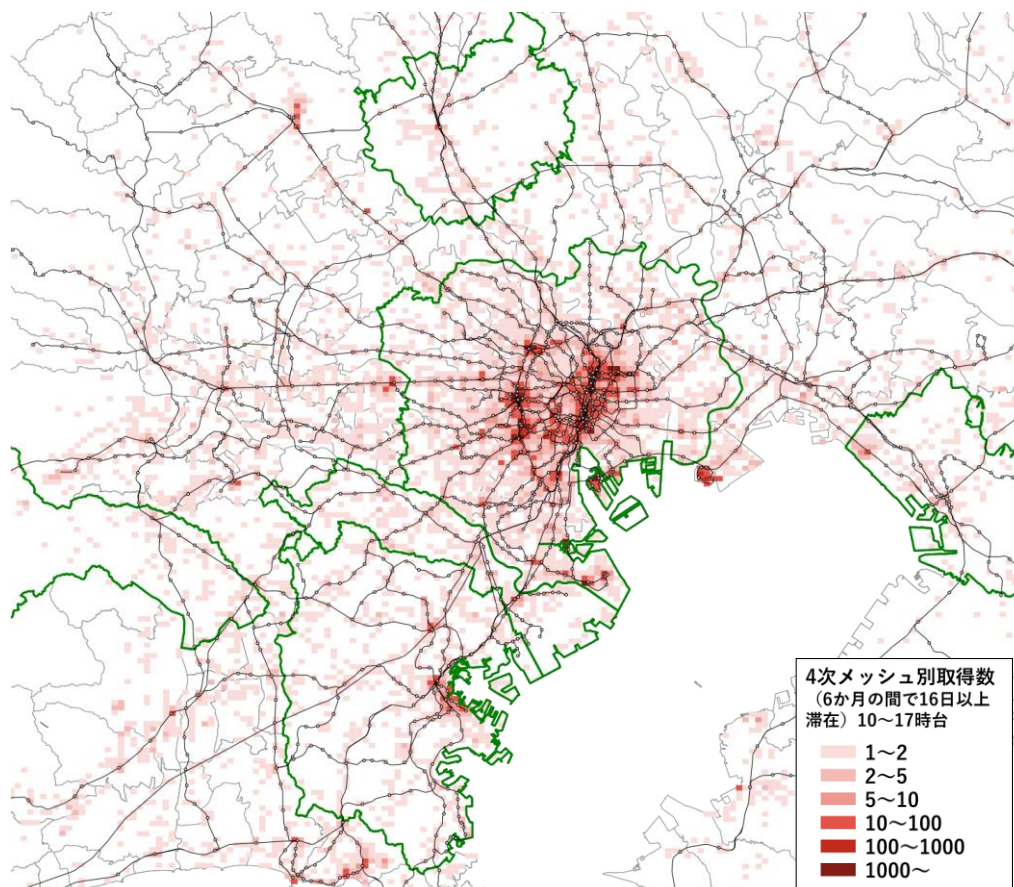
図 2-30 外国人の滞在場所
