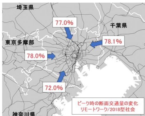
図 3-25 鉄道のピーク時の断面交通量の変化（左）と輸送密度の変化（右）
