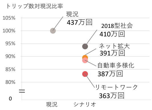
図 4-22 バストリップ数の変化
