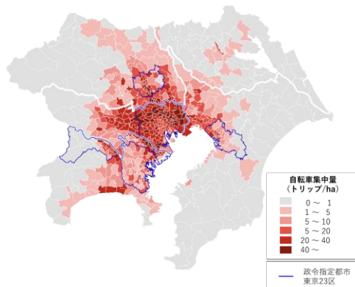
図 2-43 自転車トリップ集中量 (端末含む)
