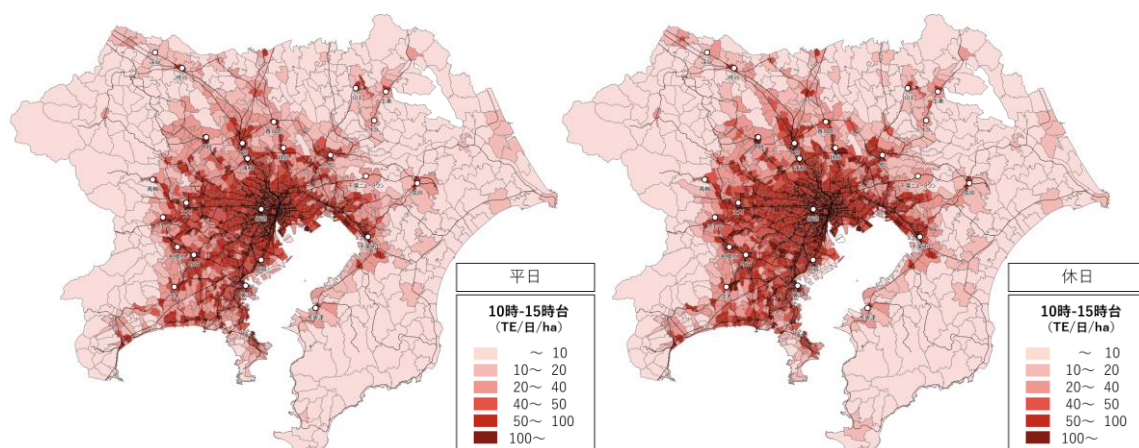
図 2-28 都市圏内居住者の集中交通量
