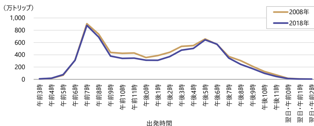
図 2-51 東京区部への時間帯別の鉄道トリップ数の変化
