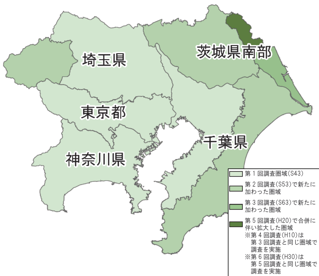
図 1-2 各調査年の対象圏域
