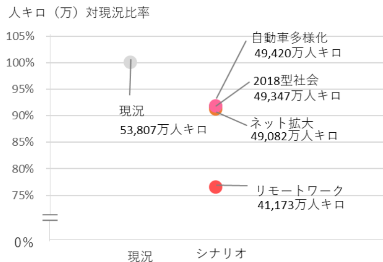
図 4-20 鉄道の乗車人キロの変化
