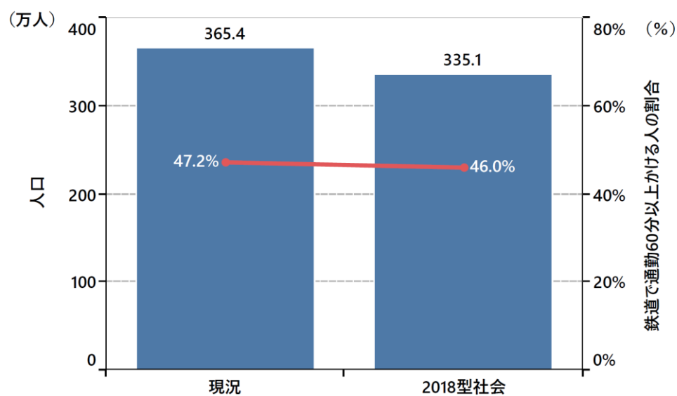
図 3-17 鉄道で通勤 60 分以上の人数の変化
