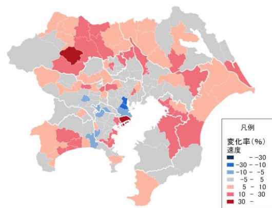
図 4-12 自動車の平均速度の変化
