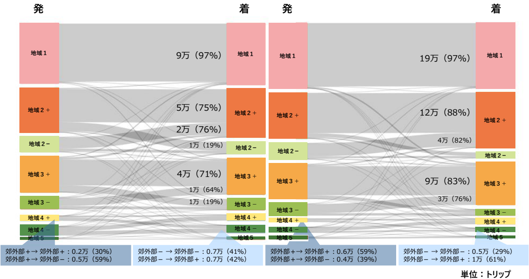
図 2-42 バスによる目的別の地域間流動（左：通勤、右：私事）
