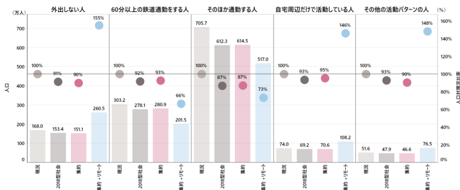
図 5-13 アクティビティパターン毎の就業者数の変化
