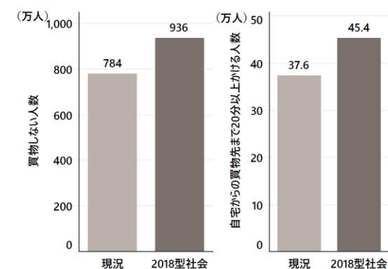
図 4-3 買物に関する高齢者の活動の変化
