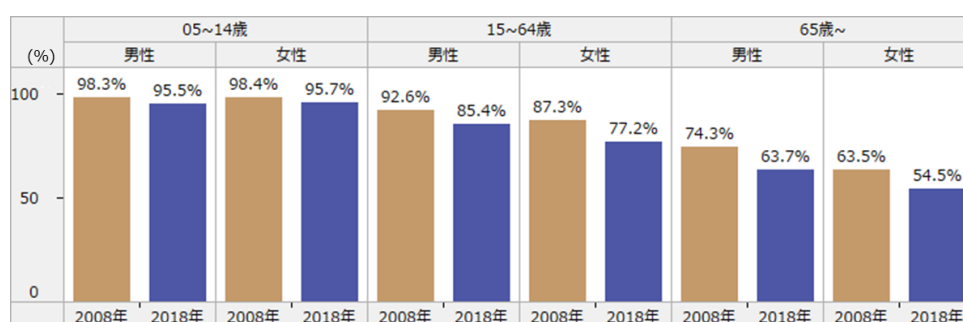
図 2-55 年齢階層別の外出率の変化
