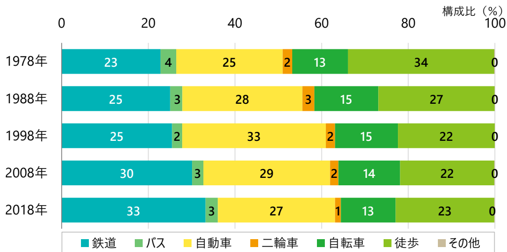
図 2-15 代表交通手段構成比の推移
