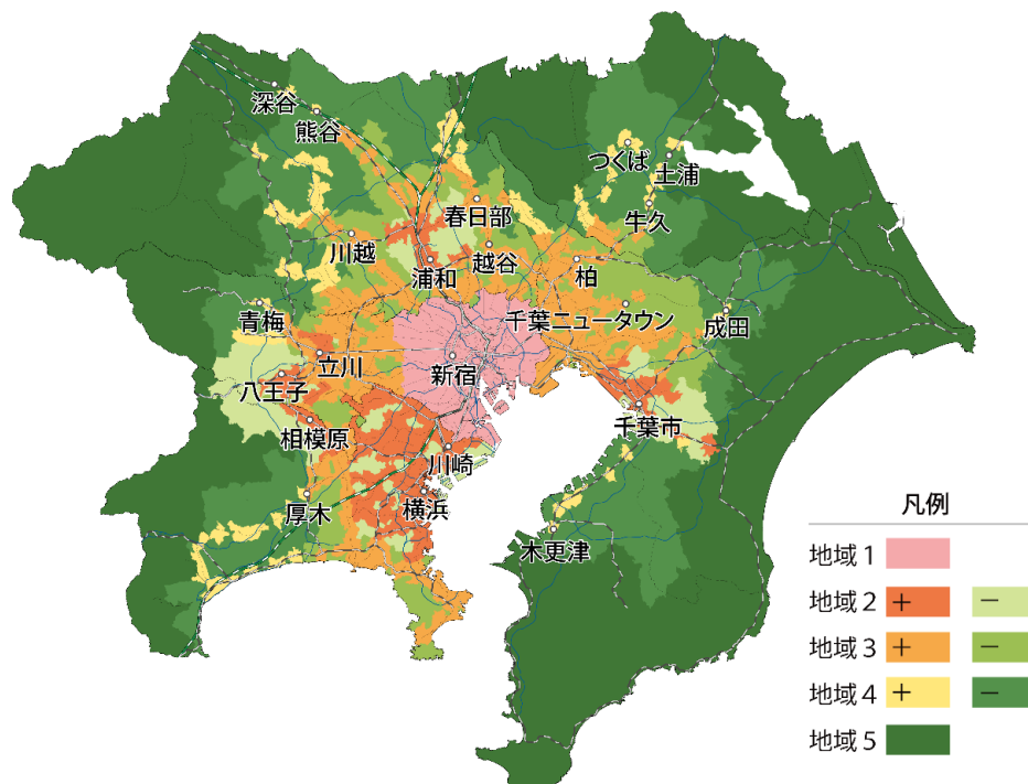
図 2-1 地域区分の設定
