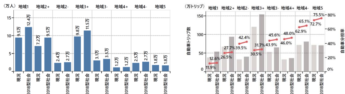
図 3-15 買物先まで時間がかかる高齢者の変化 図 3-16 高齢者の自動車利用の変化
