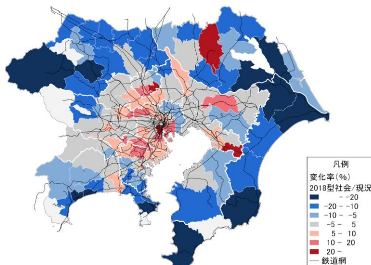
図 3-9 買物及び私事の消費金額の変化
