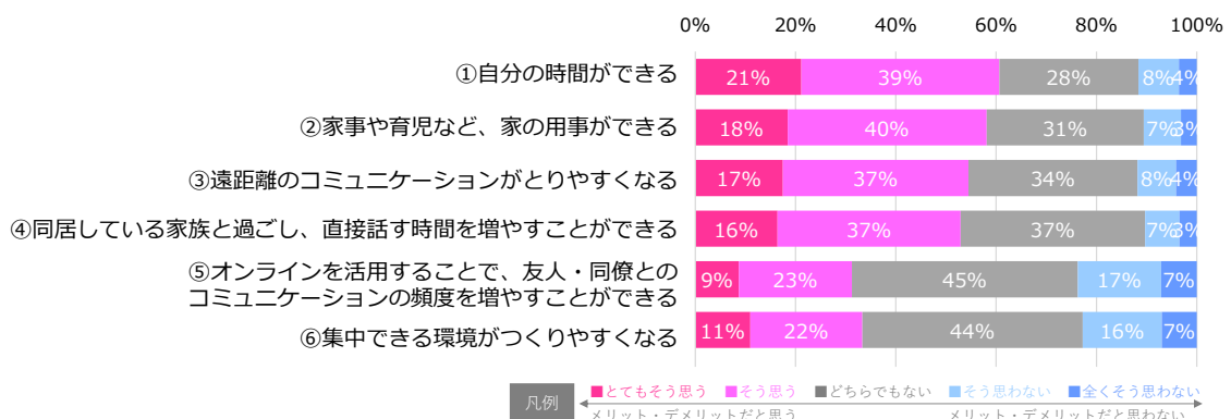
図 4-8 リモートワークに感じるメリット
