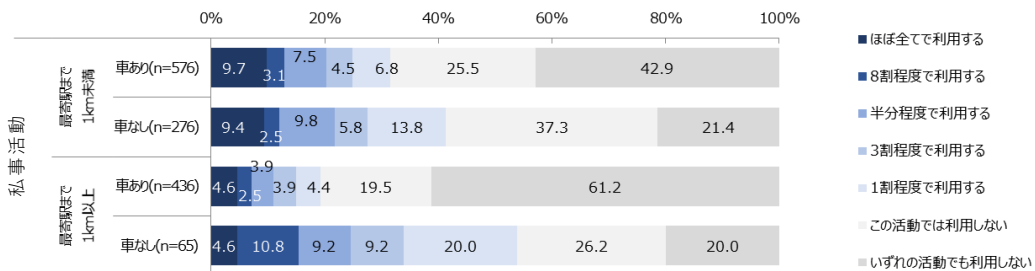
図 3-32 私事目的での自動運転の利用意向
