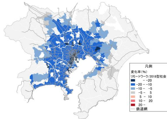
図 3-25 鉄道のピーク時の断面交通量の変化（左）と輸送密度の変化（右）
