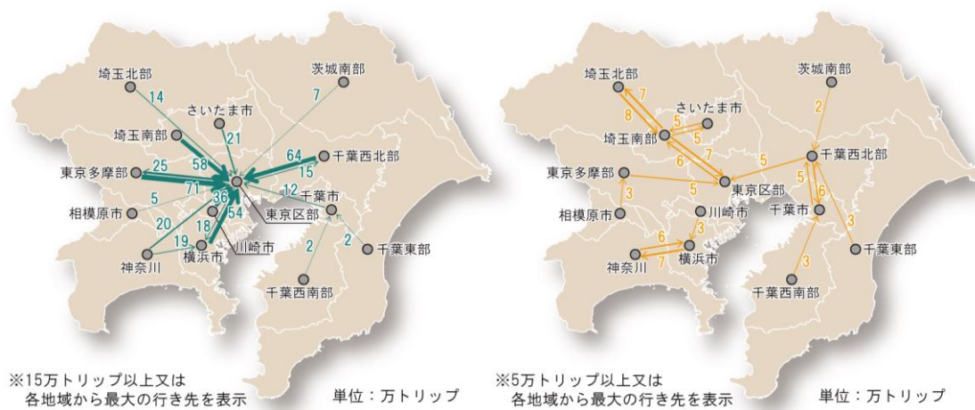
図 2-17 地域間でのトリップ数（帰宅を除く）（左：鉄道、右：自動車）
