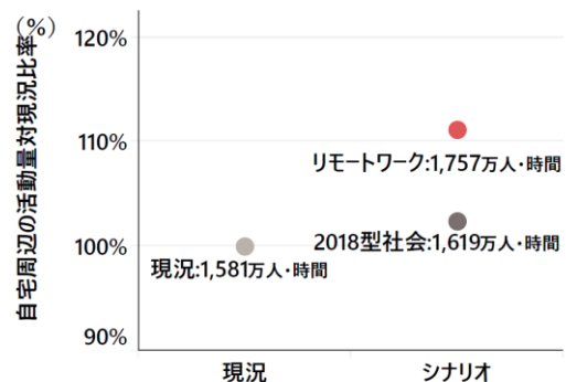
図 4-17 自宅周辺の活動時間の変化
