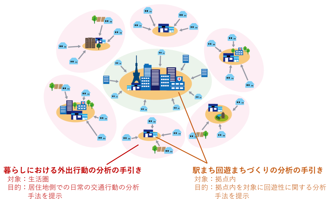
図 6-3 本書と2つの手引きの関係性
