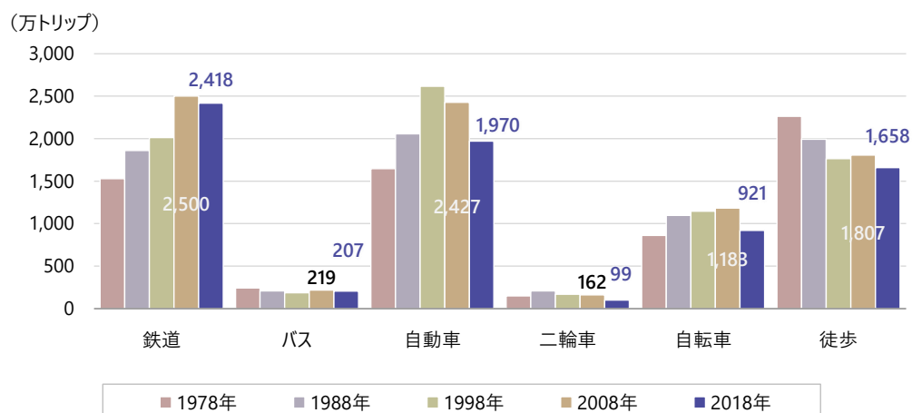
図 2-16 代表交通手段別トリップ数の推移
