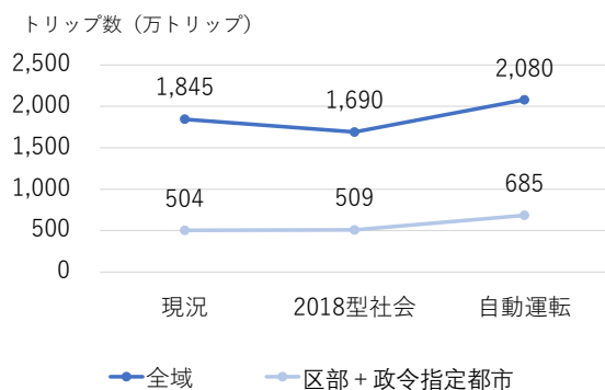
図 4-11 自動車トリップ数の変化
