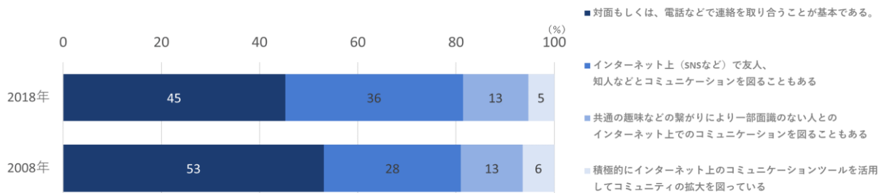
図 2-60 コミュニケーション方法の変化
