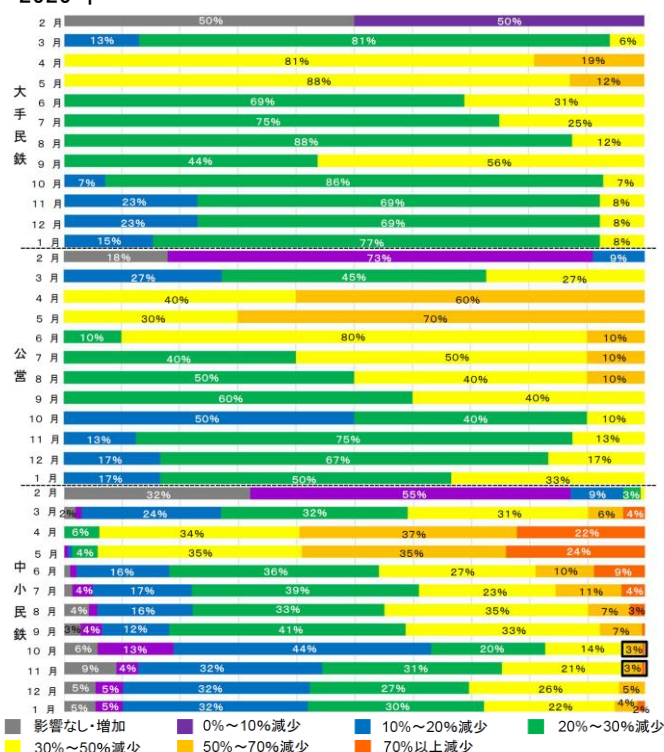
図 2-74 鉄道の輸送人員（前年同月比）
