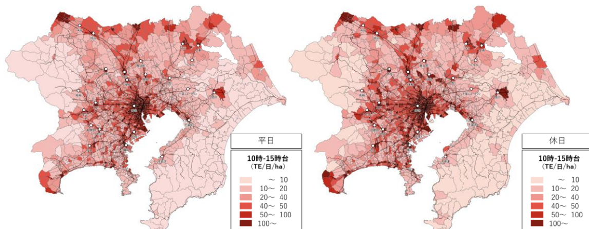
図 2-29 都市圏外居住者の集中交通量
