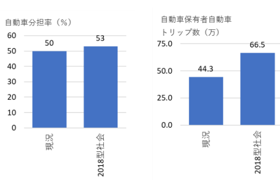
図 4-10 75 歳以上の自動車利用の変化
