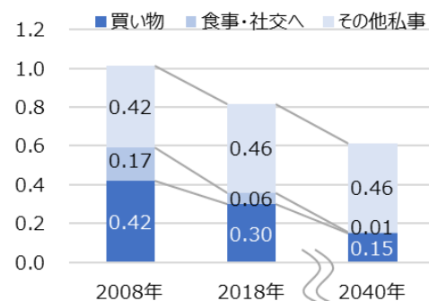
トリップ/人 高齢者・非就業
