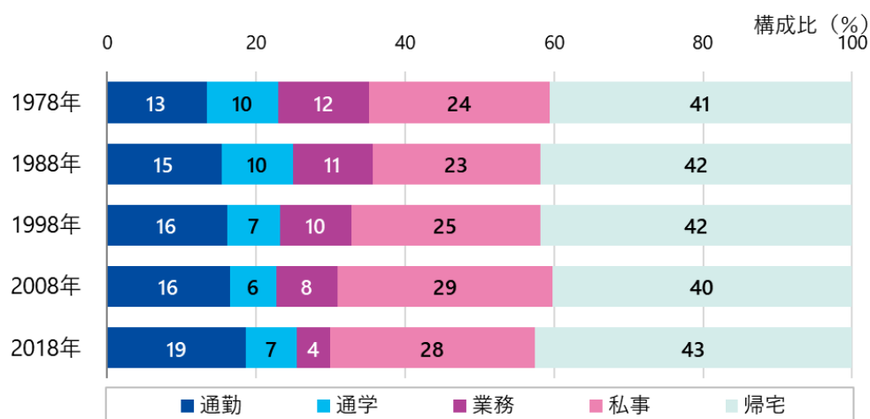
図 2-13 目的構成比の推移
