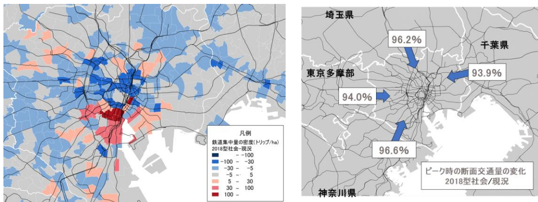
図 3-10 東京区部の鉄道集中トリップ数 (左)と東京区部境界のピーク断面交通量(右)の変化
