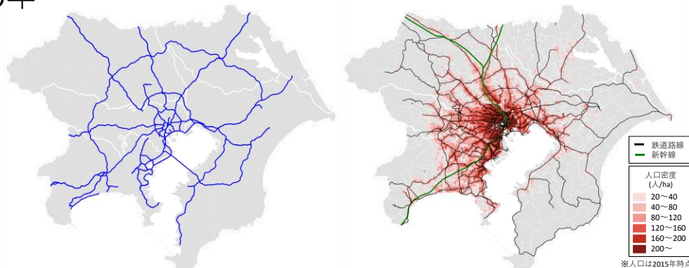
図 2-8 交通ネットワークと夜間人口の変化
