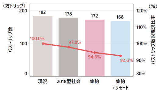
図 5-15 バストリップ数の変化
