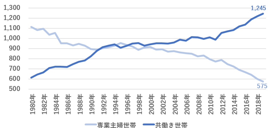
図 2-6 専業主婦世帯数と共働き世帯数の推移
