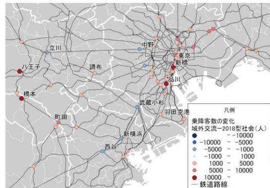
図 4-19 乗降客数の変化
