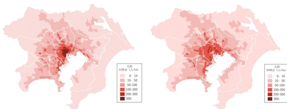
図 4-26 滞留人口の分布（左：12 時台、右：24 時台）
