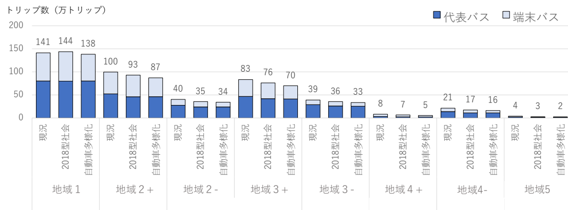
図 3-21 バストリップ数の変化
