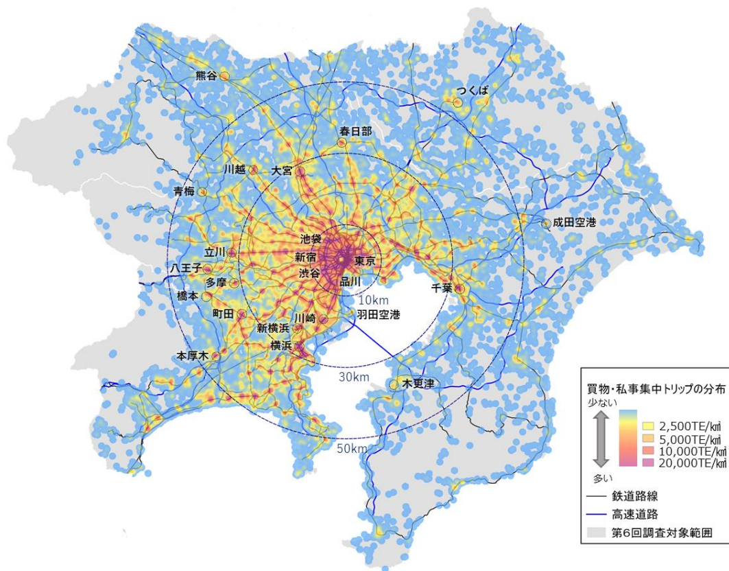
図 2-22 買物・私事集中トリップの分布
