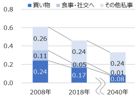
トリップ/人 高齢者・就業
