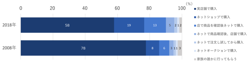
図 2-59 買回り品の買物スタイルの変化
