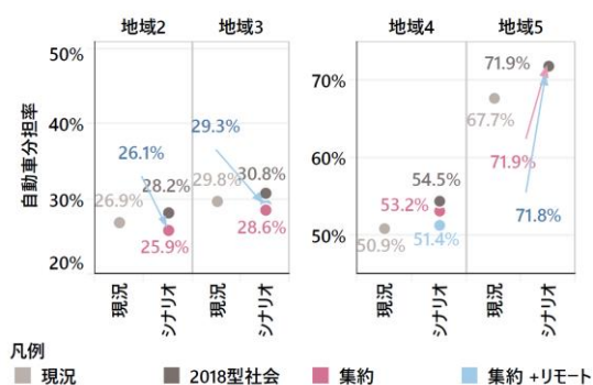
図 5-9 駅勢圏外の外出しない高齢者の変化 図 5-10 後期高齢者の自動車利用の変化
