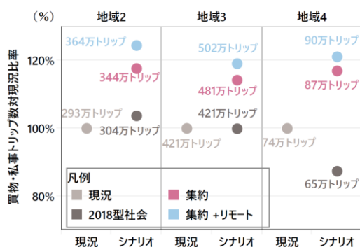
図 5-11 駅勢圏内の買物・私事トリップ数の変化
