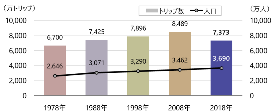
図 2-9 総トリップ数と総人口の推移
