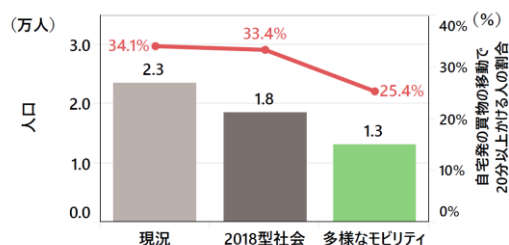
図 5-3 高齢者の私事トリップ数の変化 図 5-4 買物に 20 分以上かける人口の変化
